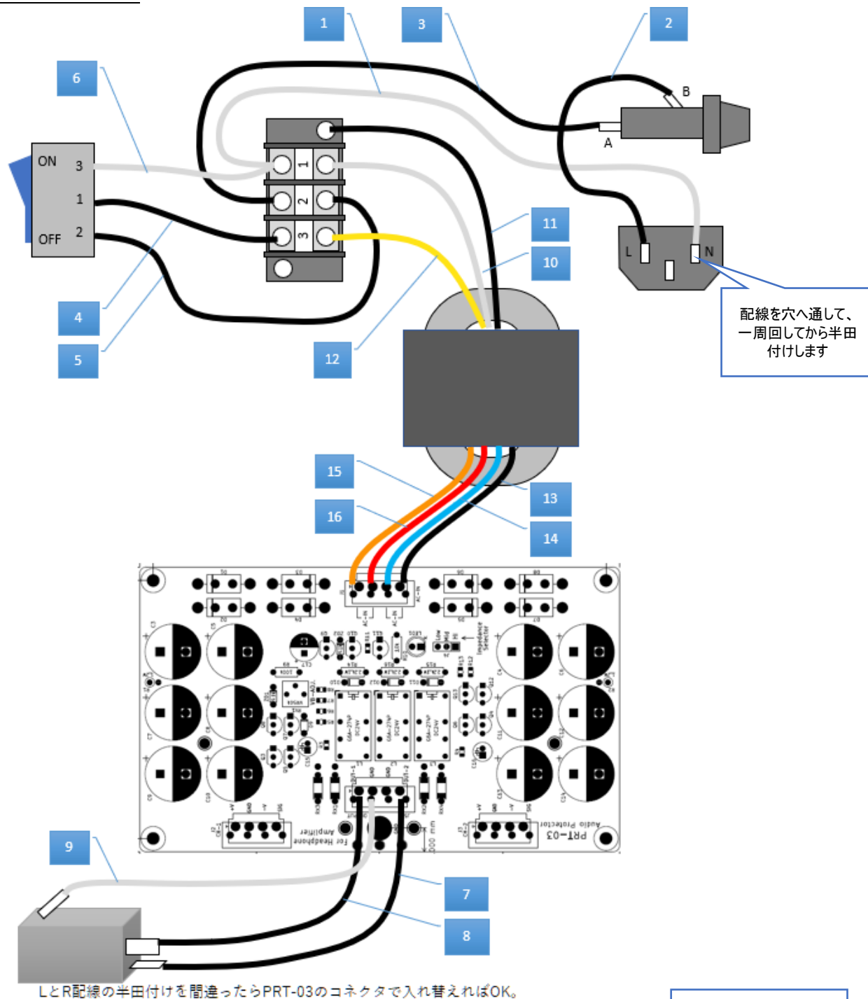
配線図－ 1 （太い配線部分）
