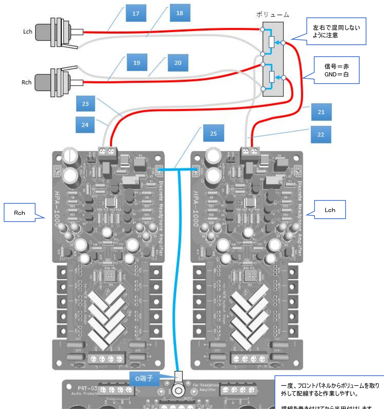
配線図－２（オーディオ信号配線）
